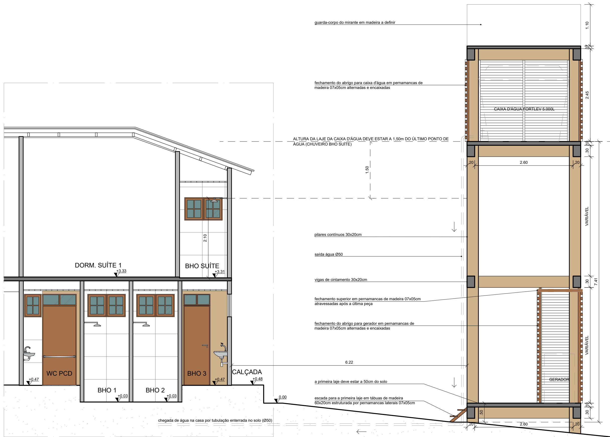
MÓDULO CAIXA D'ÁGUA - CORTE ESQUEMÁTICO ESC: 1:50
